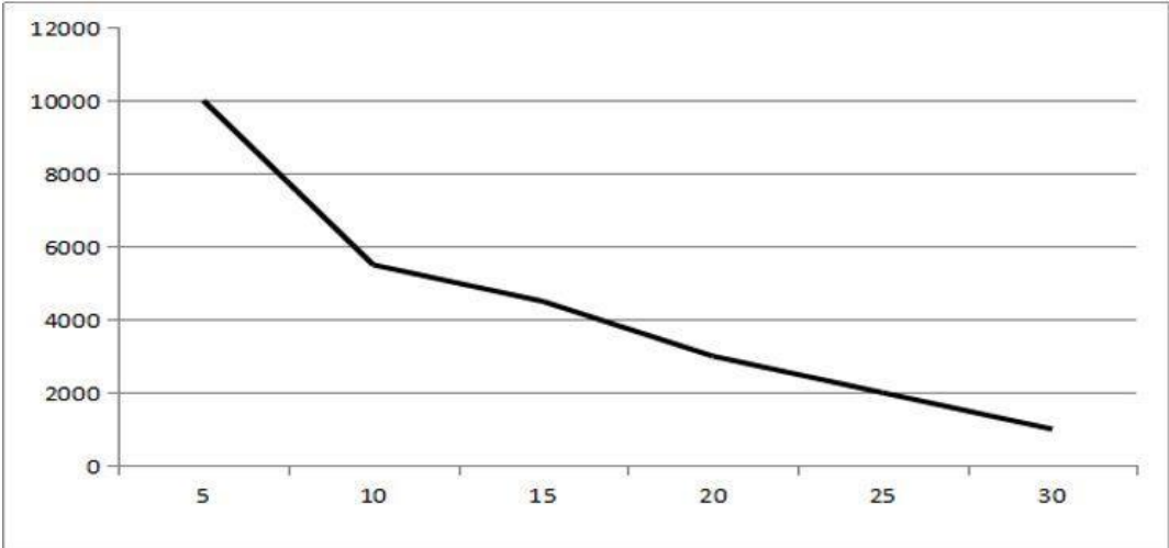
图 2-1 建筑物平均高度的变化对基站覆盖范围的影响
