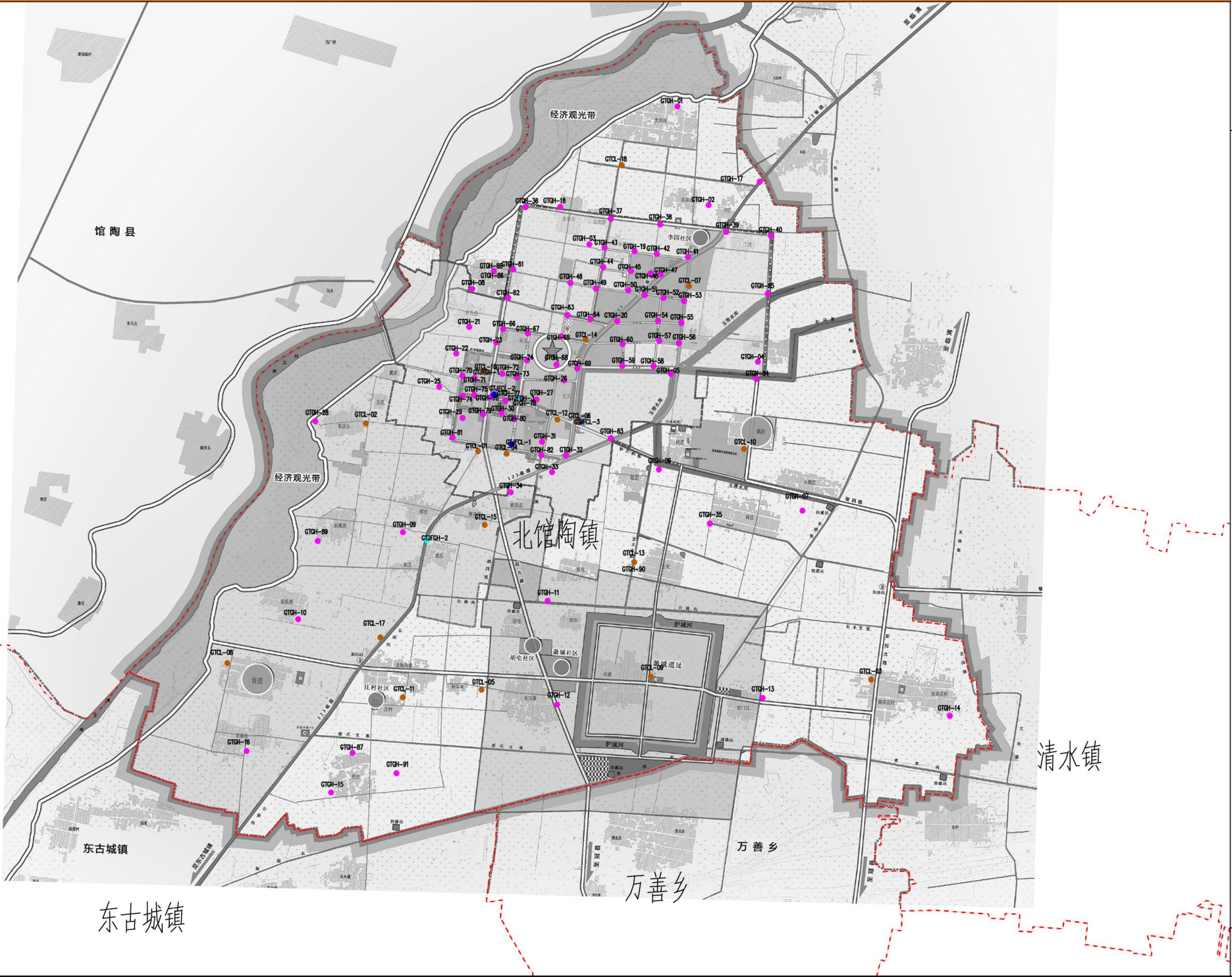
北馆陶镇规划基站站点和机房分布图
