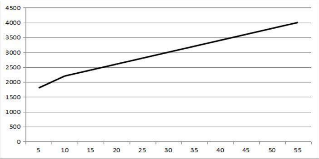
图 2-2 建筑物平均间距的变化对基站覆盖范围的影响
