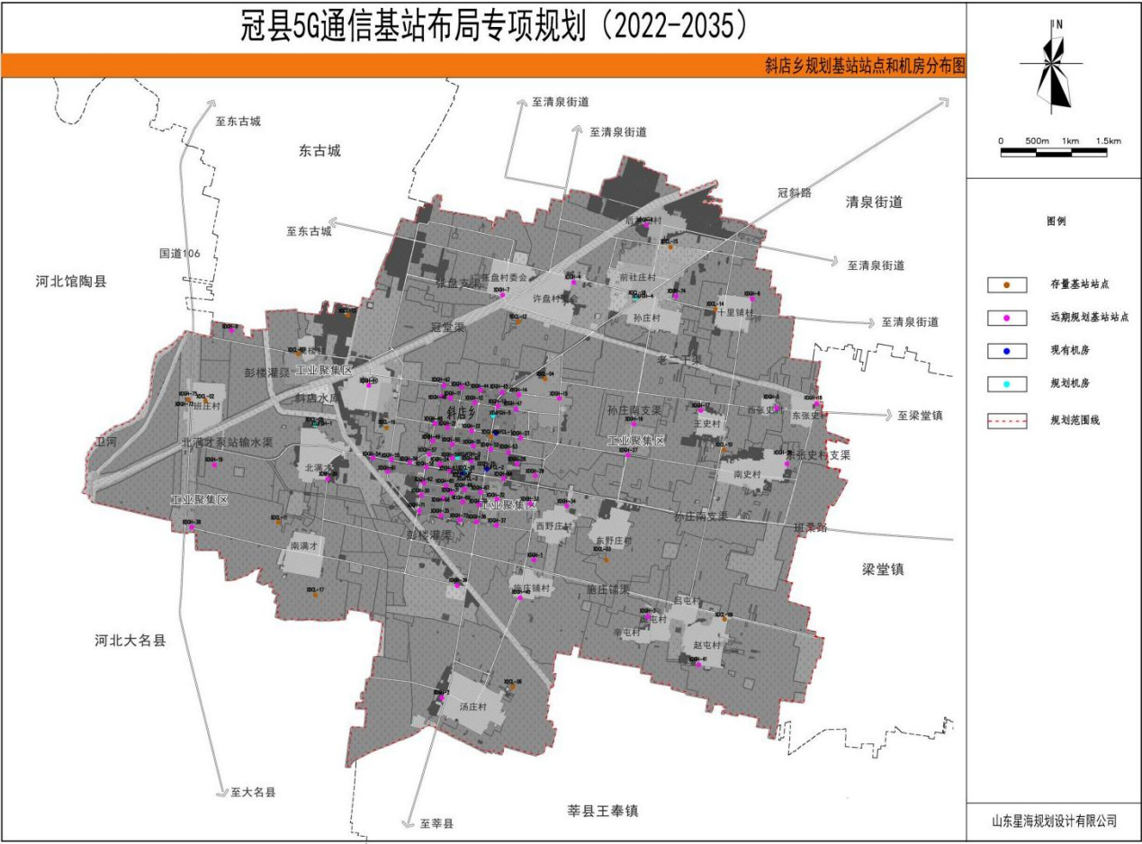
图 3-16 斜店乡规划基站分布图
