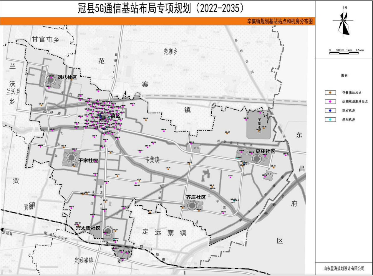
图 3-15 辛集镇规划基站分布图
