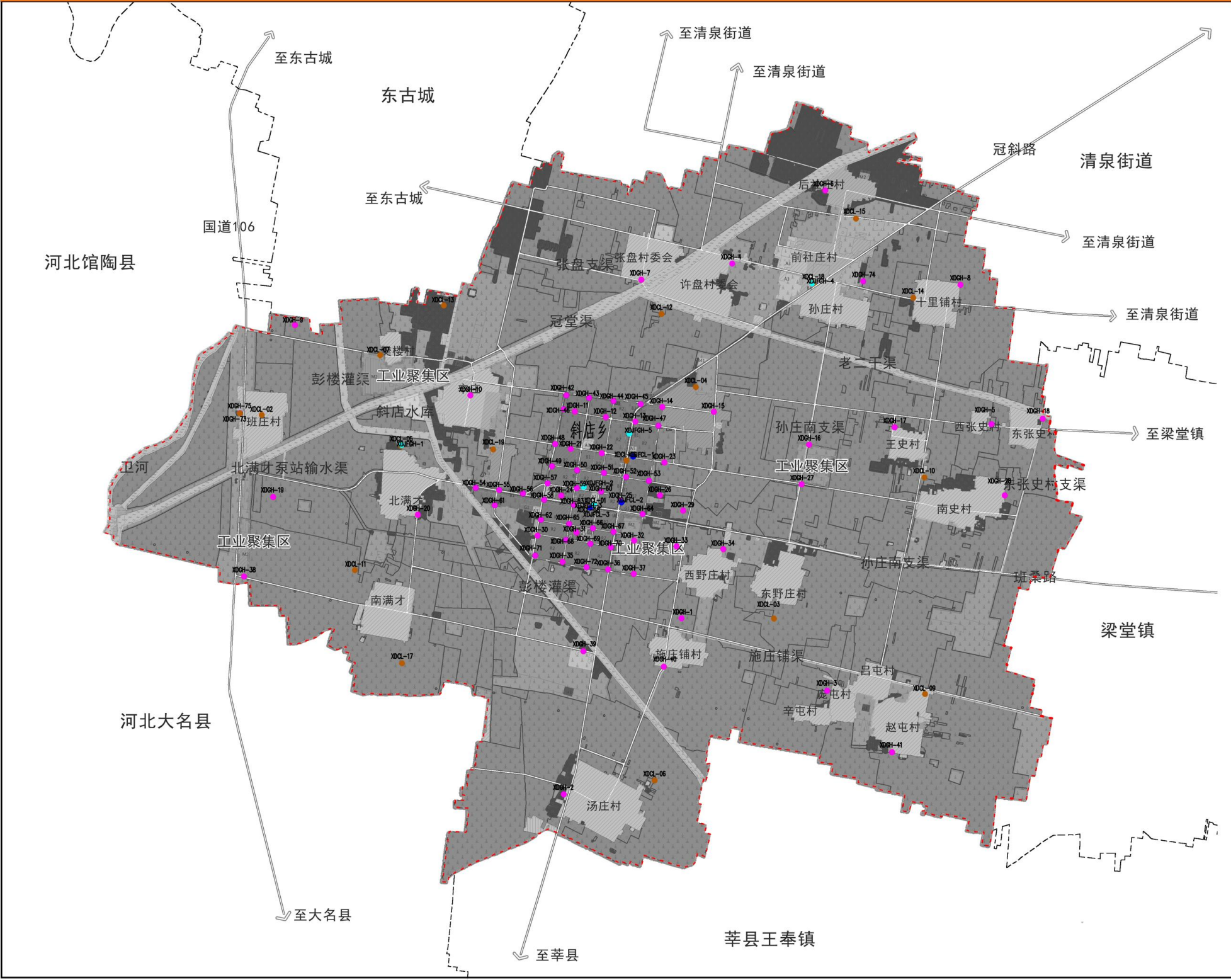
斜店乡规划基站站点和机房分布图
