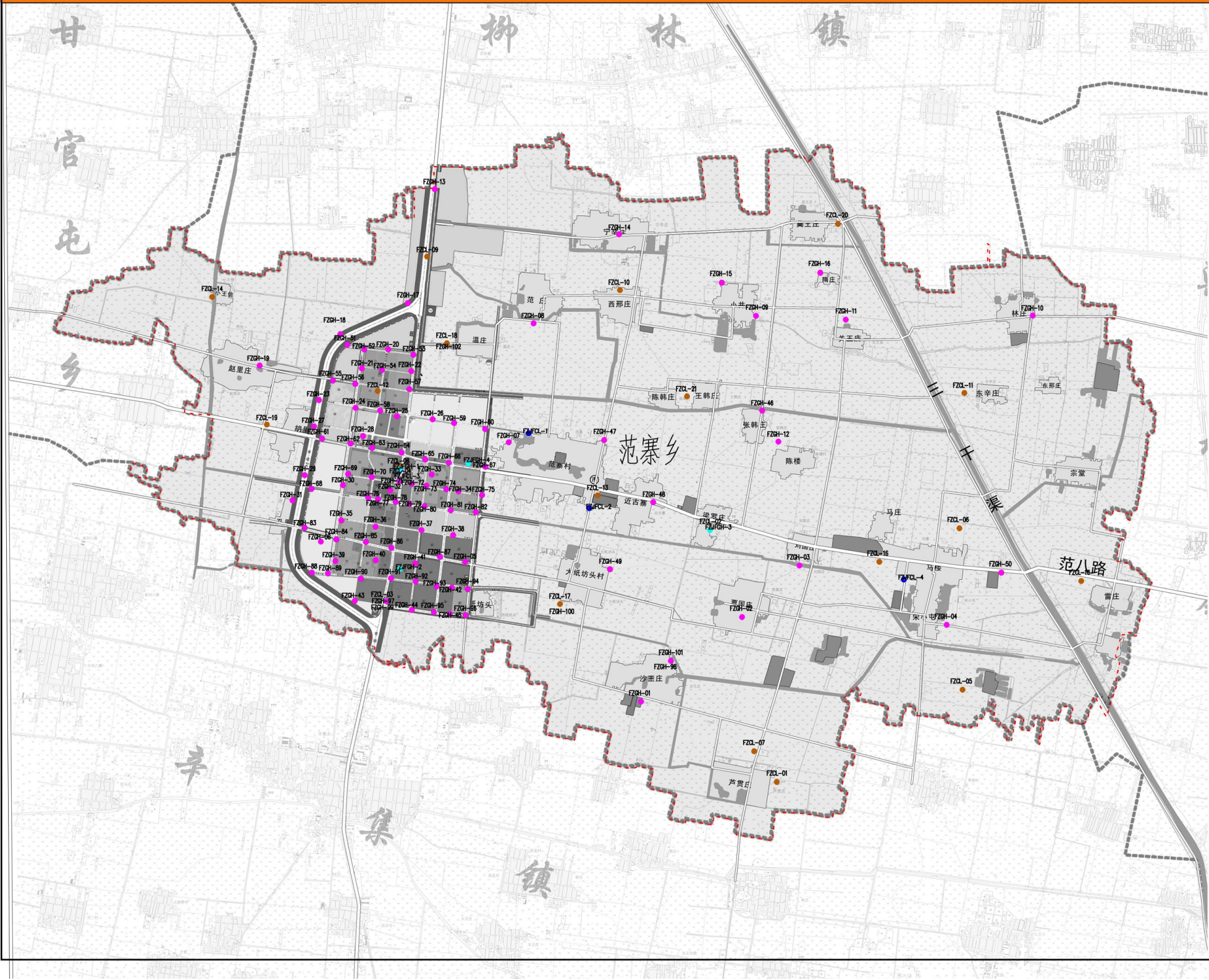
范寨乡规划基站站点和机房分布图
