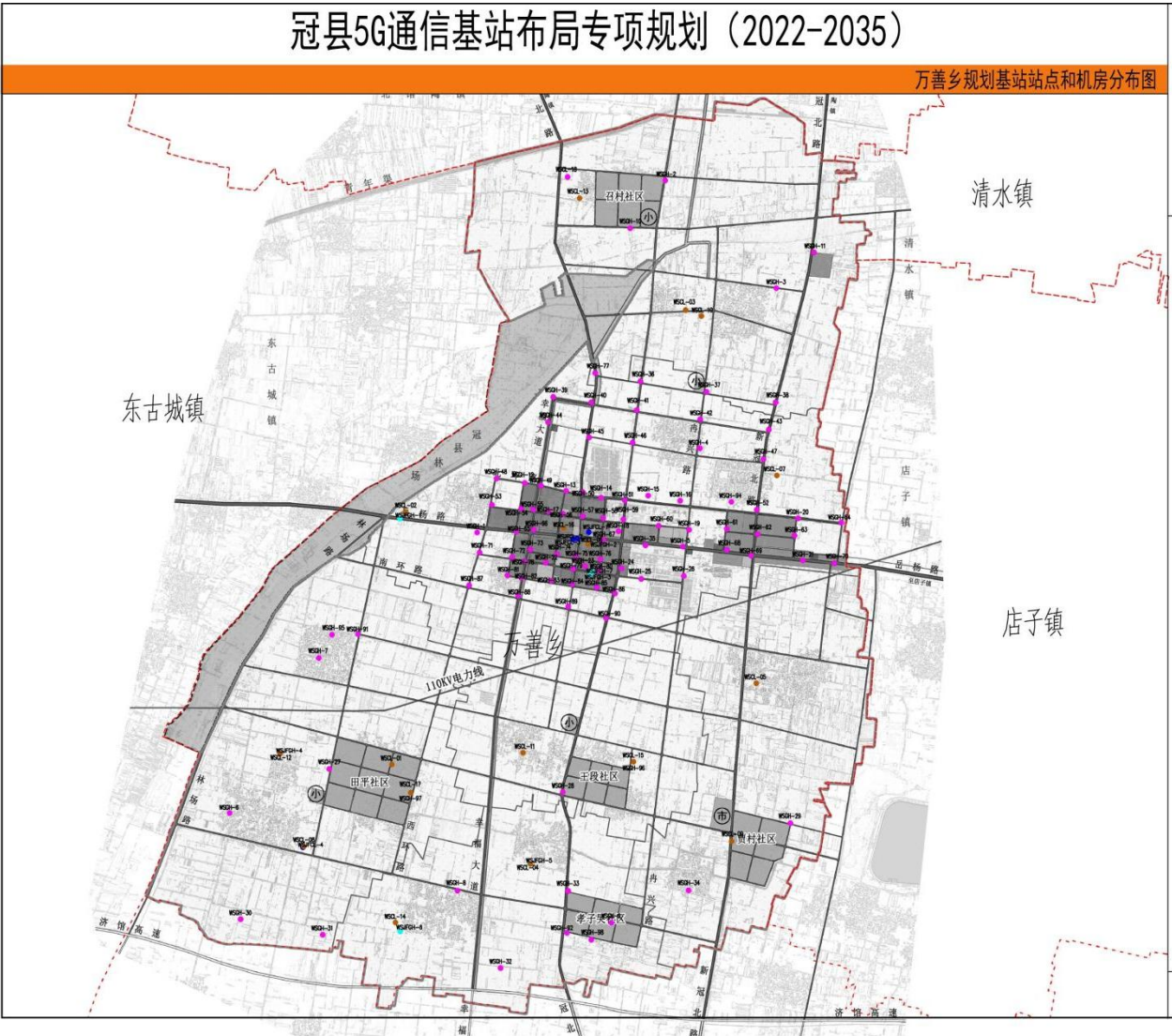
图 3-10 万善乡规划基站分布图
