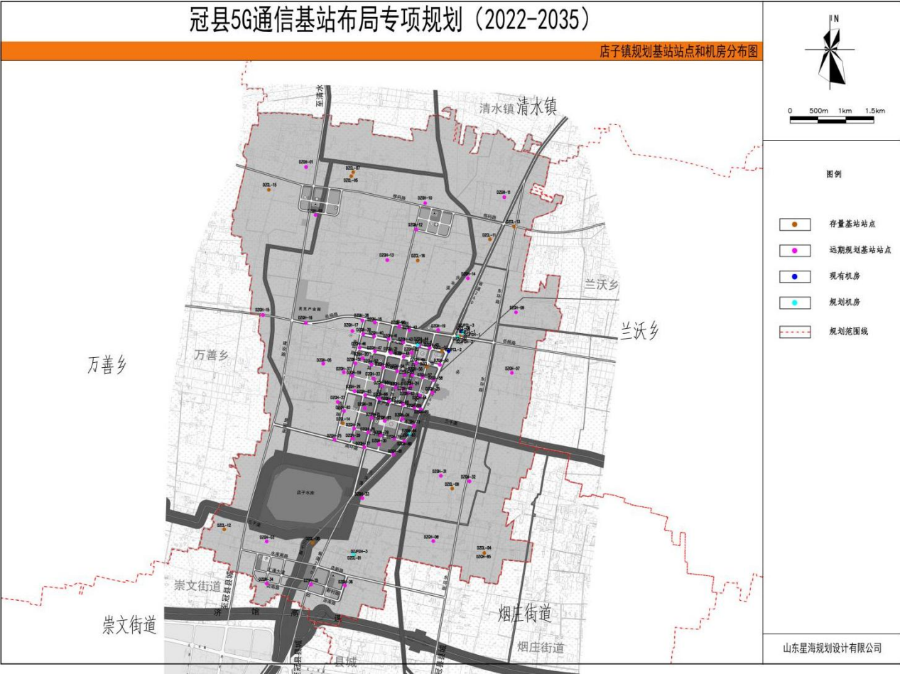
图 3-11 店子镇规划基站分布图
