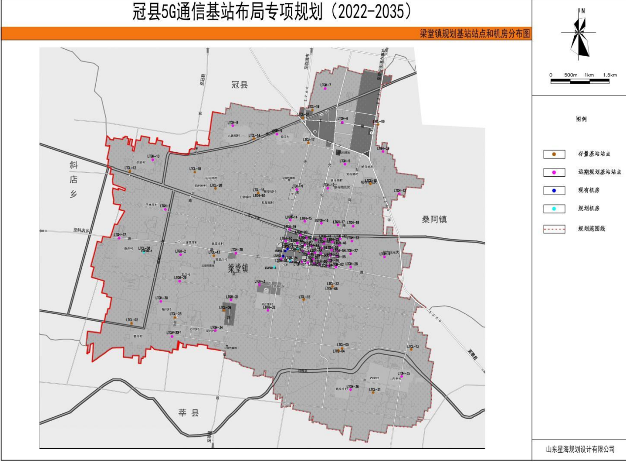
图 3-17 梁堂镇规划基站分布图
