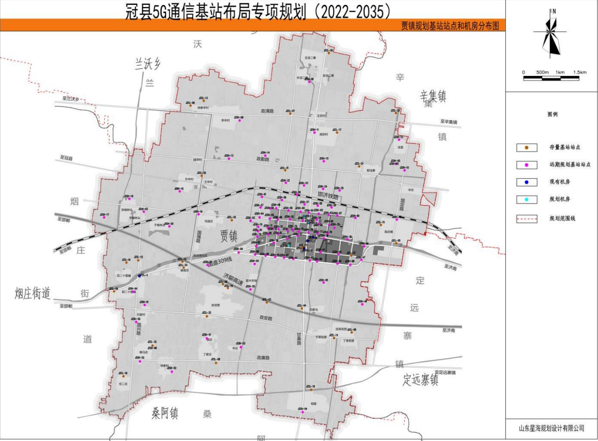
图 3-14 贾镇规划基站分布图
