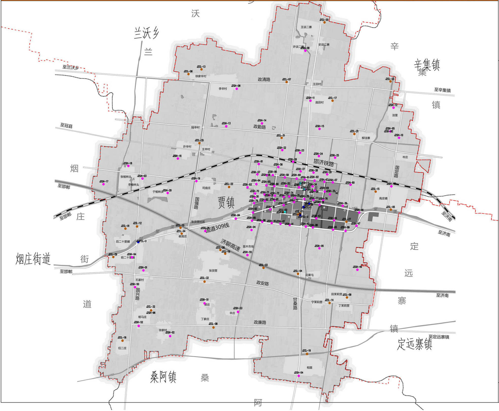
贾镇规划基站站点和机房分布图
