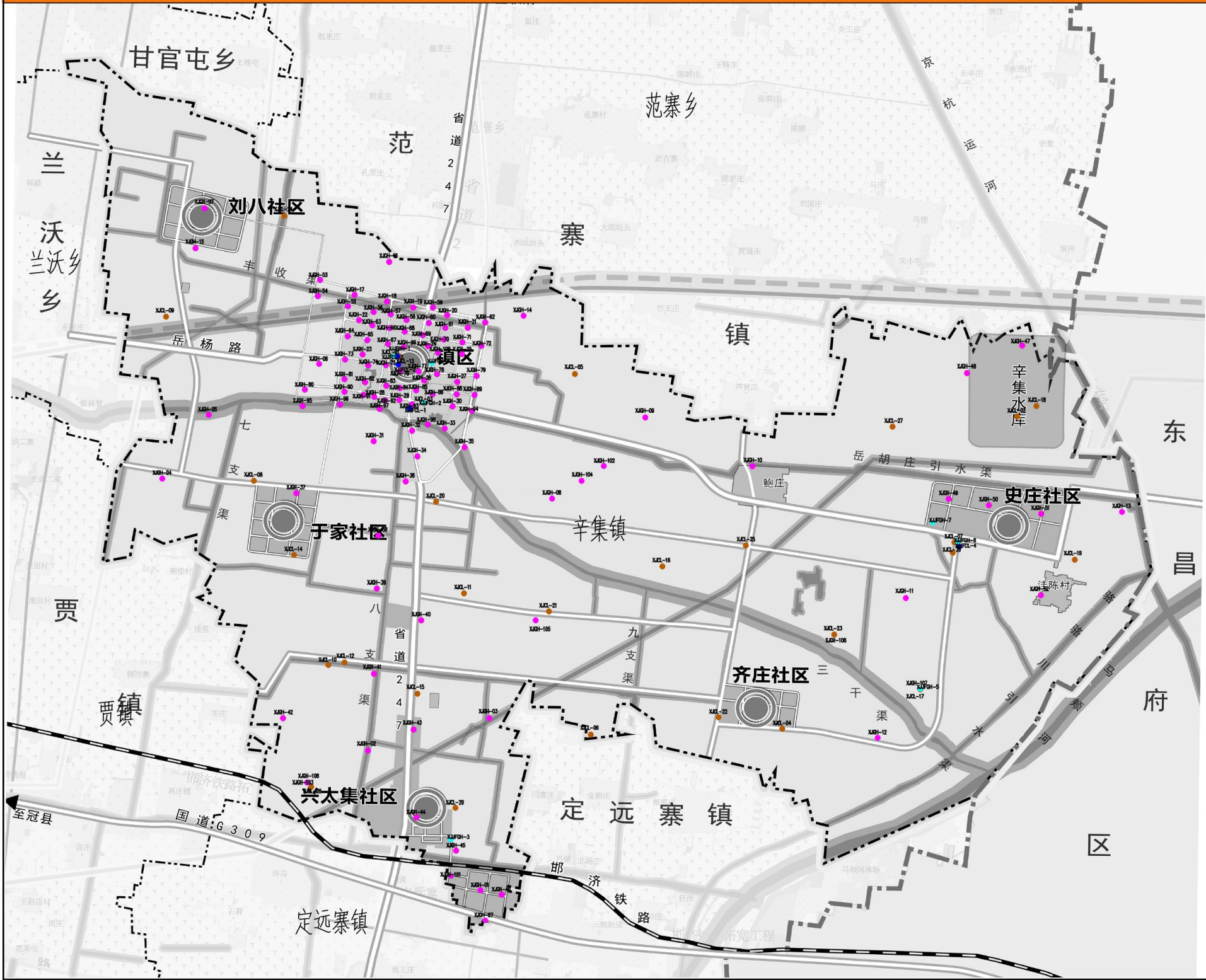
辛集镇规划基站站点和机房分布图
