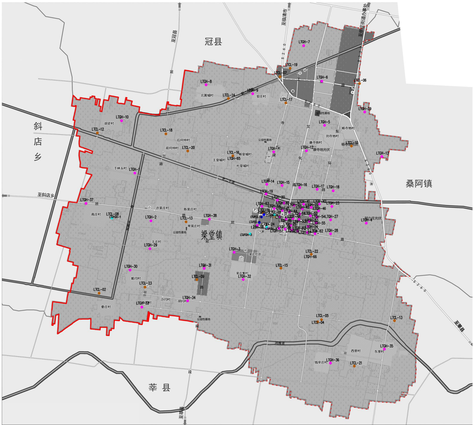
梁堂镇规划基站站点和机房分布图
