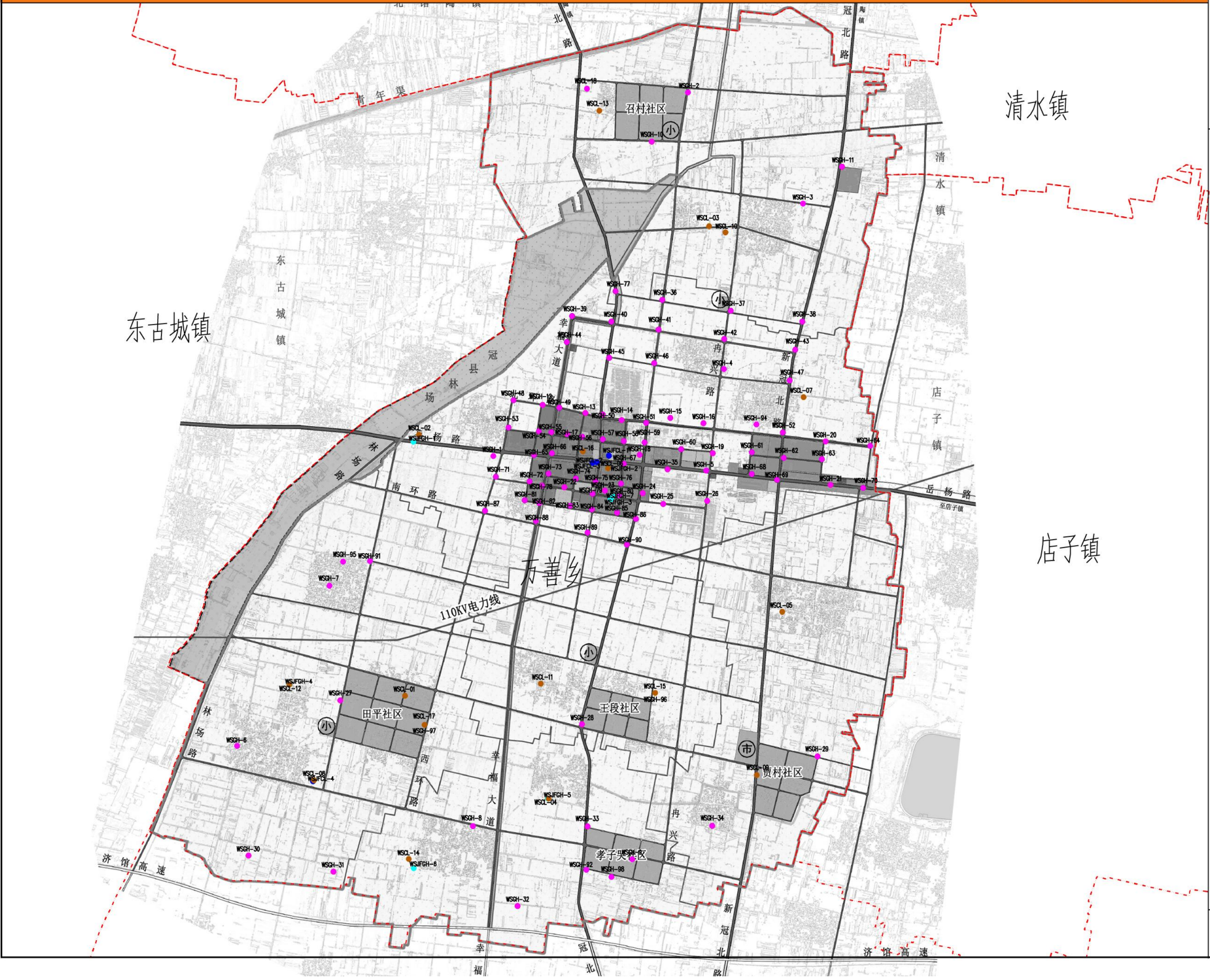
万善乡规划基站站点和机房分布图
