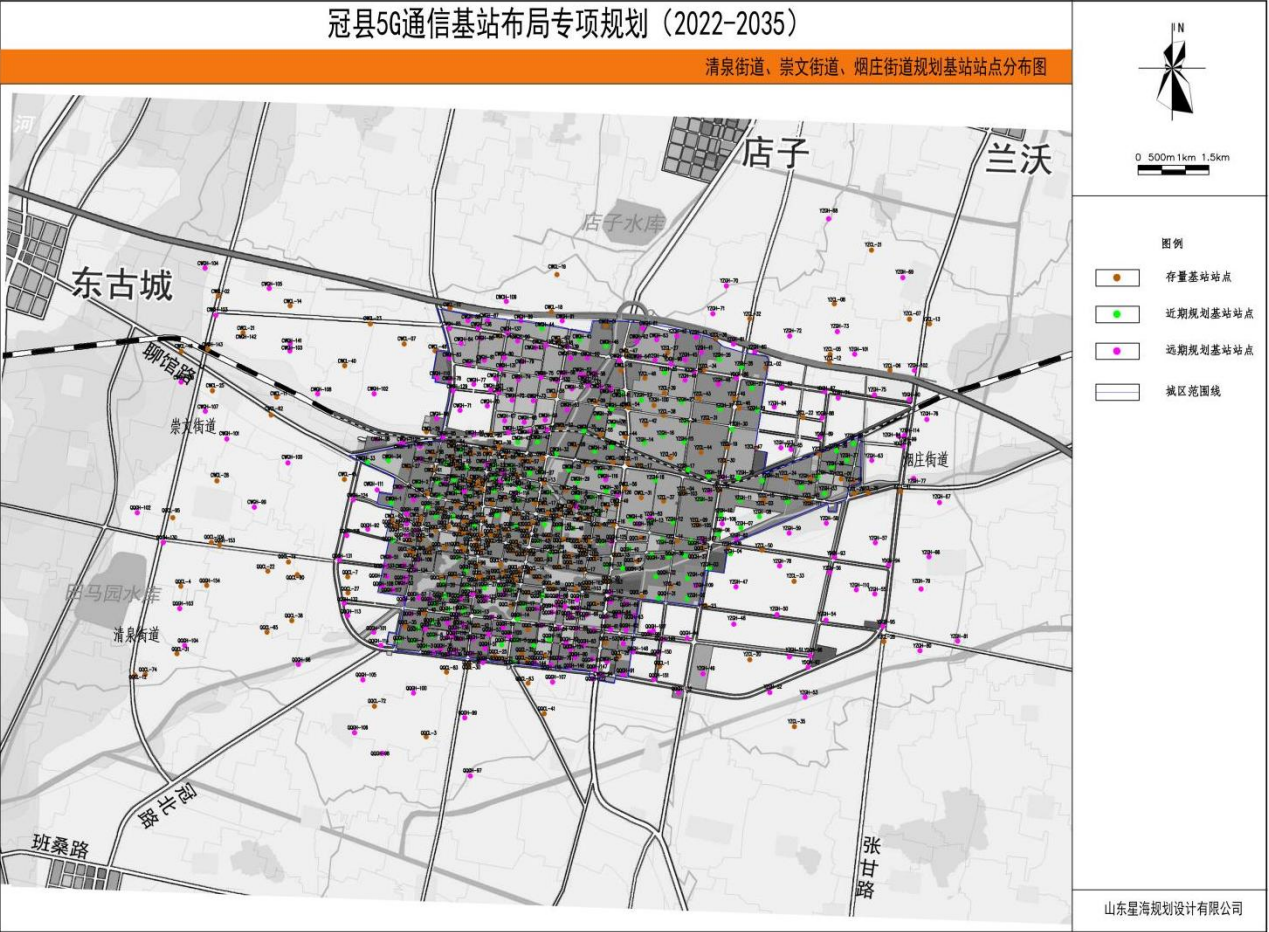
图 3-20 清泉街道 崇文街道 烟庄街道规划基站分布图
