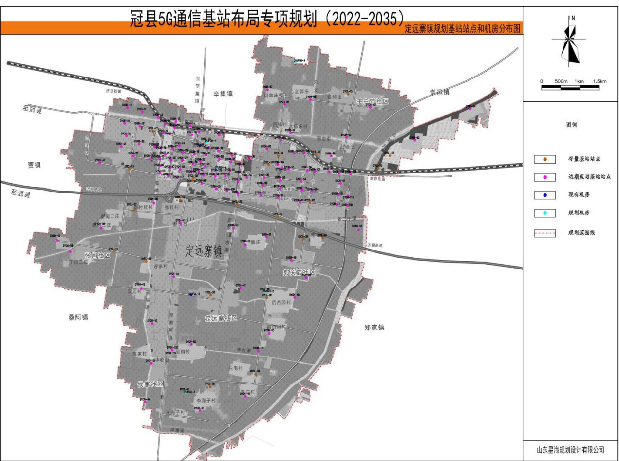
图 3-19 定远寨镇规划基站分布图
