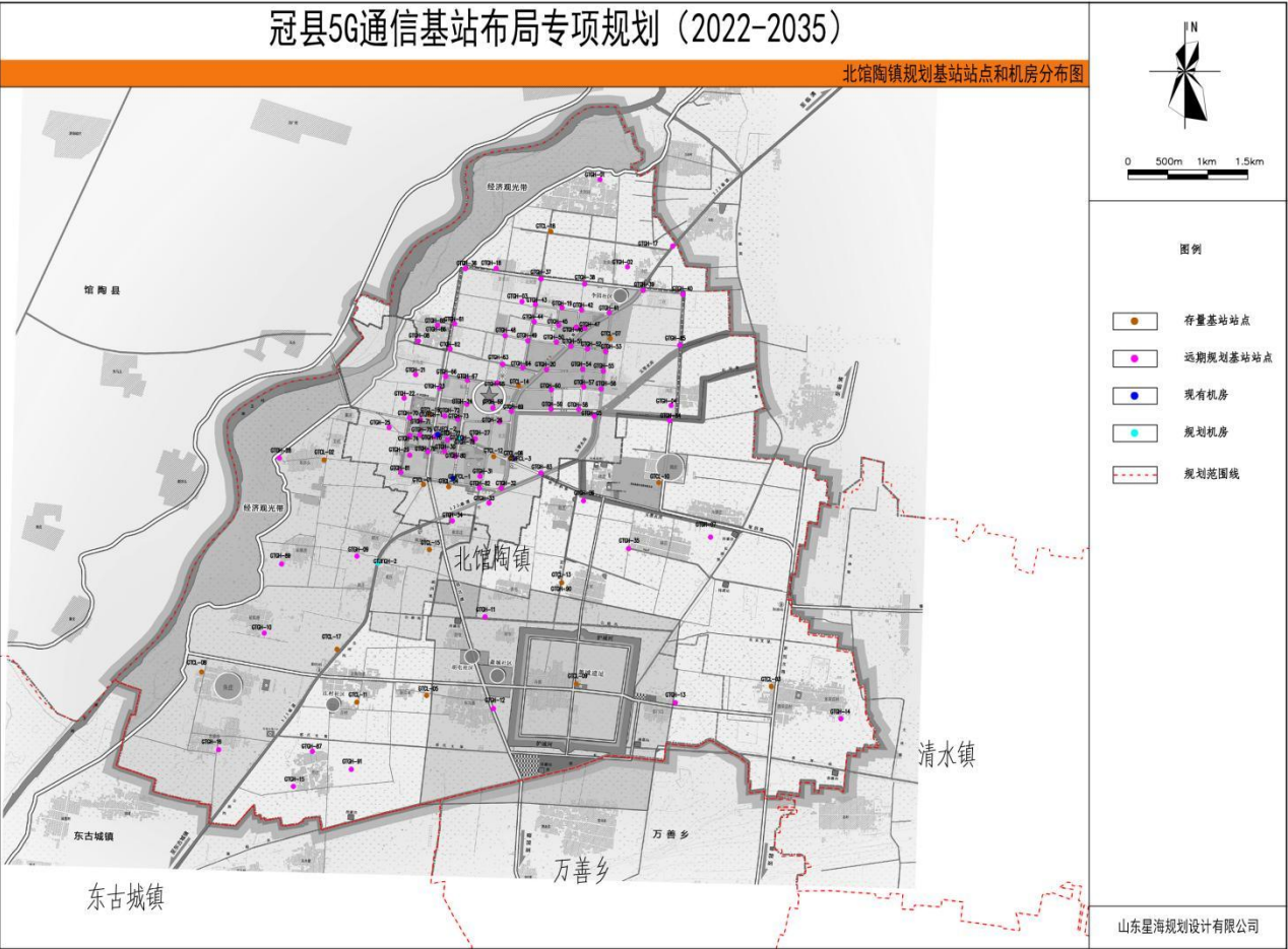
图 3-5 北馆陶镇规划站点分布图
